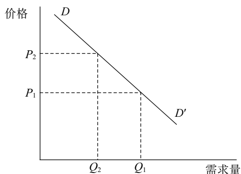
图 1-1 需求曲线
